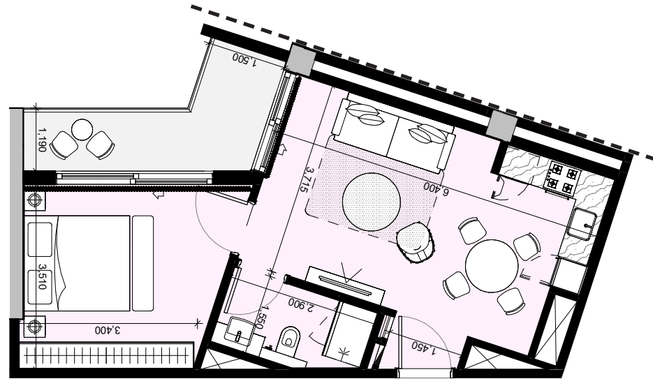
1 BEDROOM TYPE 03 55.17 m 2
